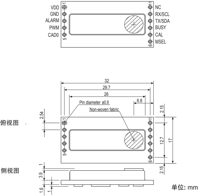
引脚配置
