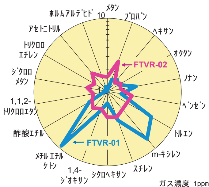
図 FTVR-02の各種ガス検知特性（FTVR-01との比較）
