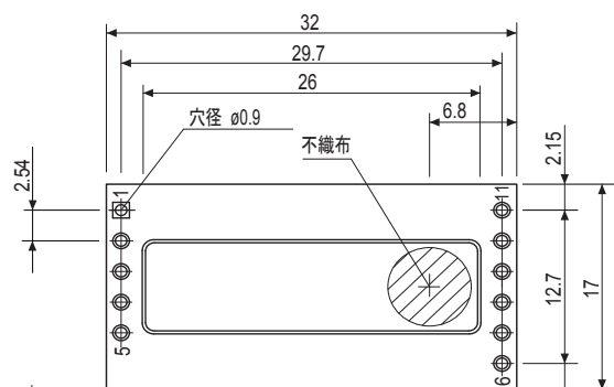
上面図
