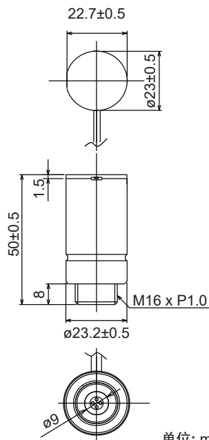
KE-12F3LF / KE-25F3LF / KE-25F3LFM (threaded top)
