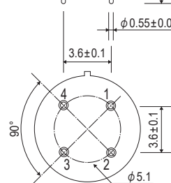
仰视图
