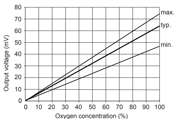
Fig. 3a - KE-25 sensitivity characteristics
