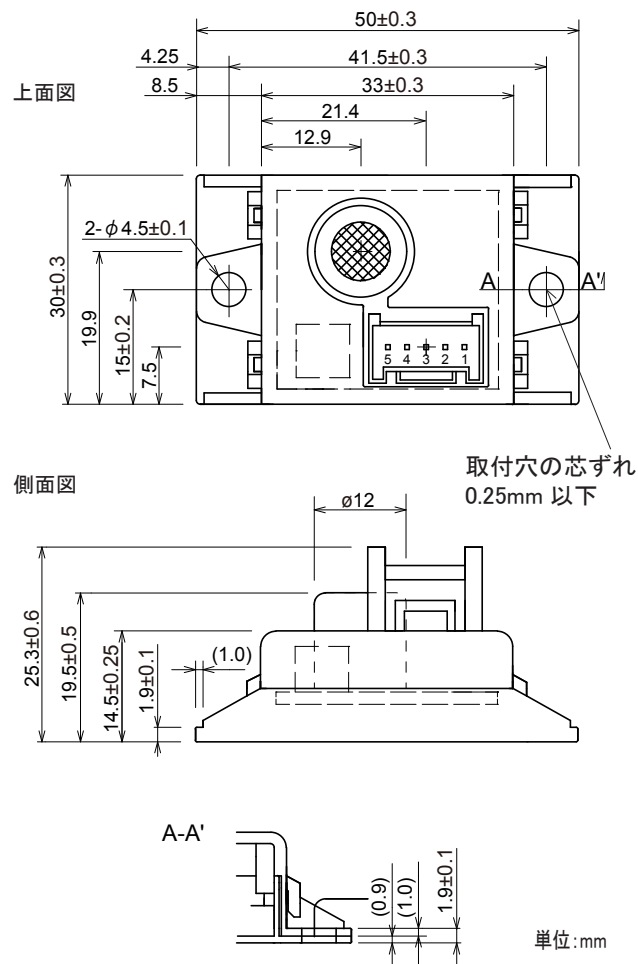
A-A' 断面 ※締め付け取付状態にて
