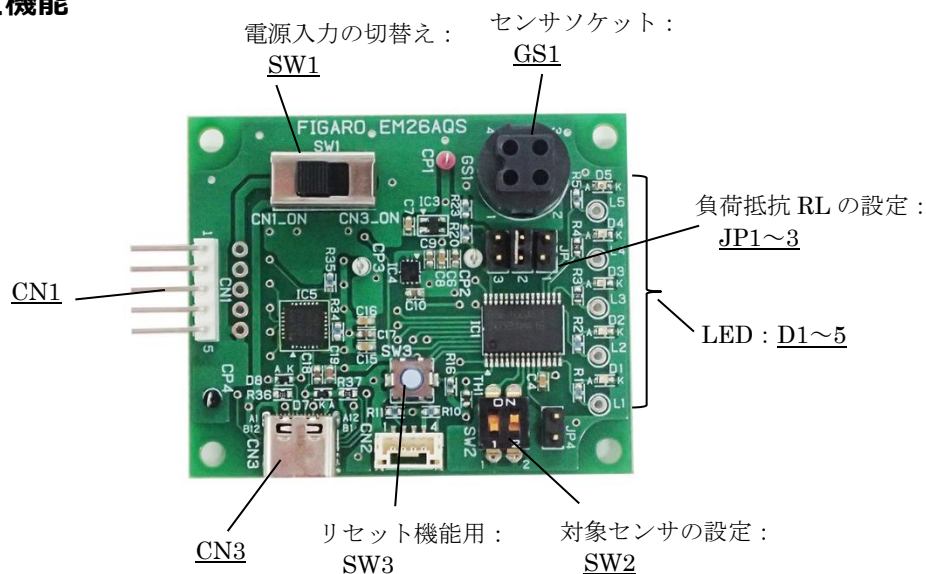
図1 各部の名称
