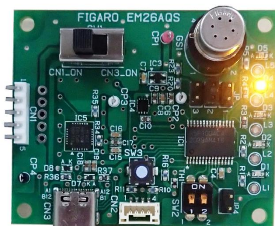
図 2 LED 点灯のイメージ (D4 点灯時)
